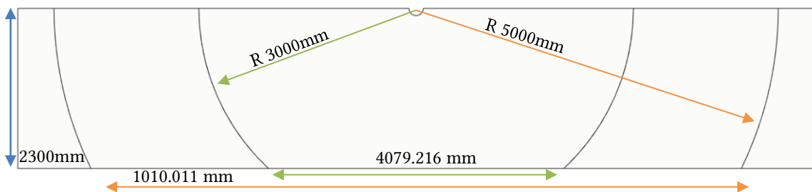
Abbildung 18: Abdeckung Infrarotbewegungsmelder bei Raumhöhe von 2.3m
